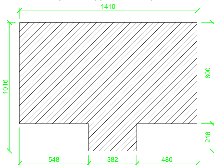
SHEMA TLOCRTA PRIZEMLJA
