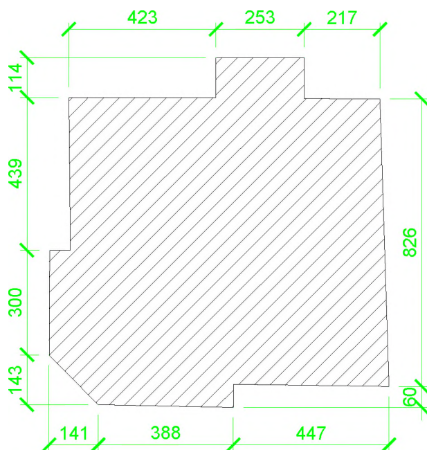
SHEMA TLOCRTA KATA
