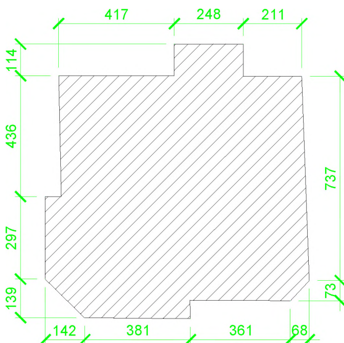
SHEMA TLOCRTA PRIZEMLJA
